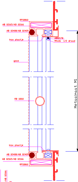
Doorsnede A-A
