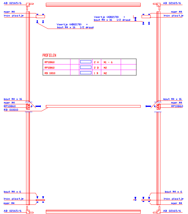
Doorsnede A-A
