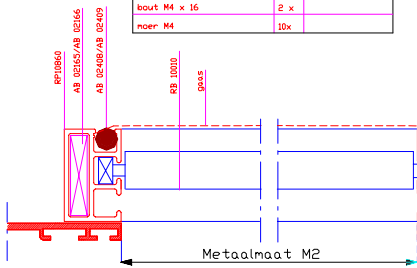
Doorsnede B-B
